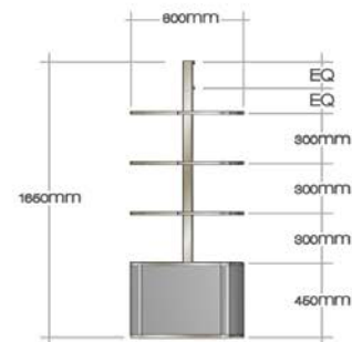
RIGHT ELEVATION
