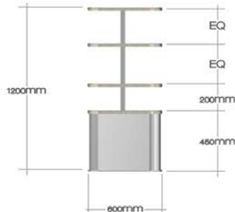
RIGHT ELEVATION
