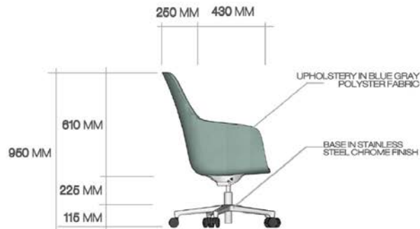
RIGHT ELEVATION
