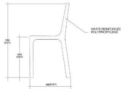
RIGHT ELEVATION
