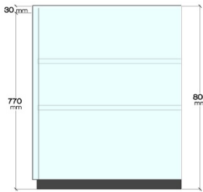
RIGHT ELEVATION
