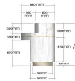
RIGHT ELEVATION
