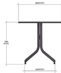
RIGHT ELEVATION
