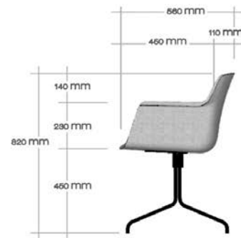
RIGHT ELEVATION
